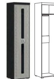
Шкаф плательный 500 x 420, h 2090
