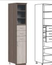
Пенал, на 400 мм, с ящиками 400 x 600, h 2100
