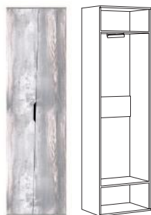
Шкаф плательный 600 x 400, h 2140
