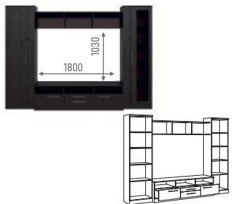
Горка 3000 x 490, h 2130
