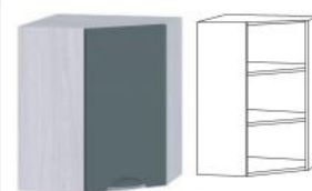
Шкаф навесн., на 600 мм угловой, с 2 полками 600 x 600, h 900
