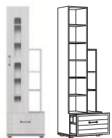
Пенал со стеклом 600 x 410, h 2120
