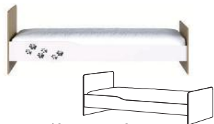
Кровать 1-сп. (сп. место 900*2000), б./матраца 2035 x 950, h 800
